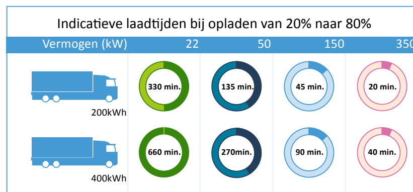
Figuur 1 Laadtijden van verschillende laadvermogens
